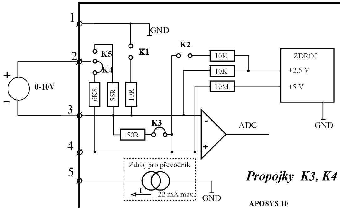
Připojení napěťového signálu 0 - 10 V
