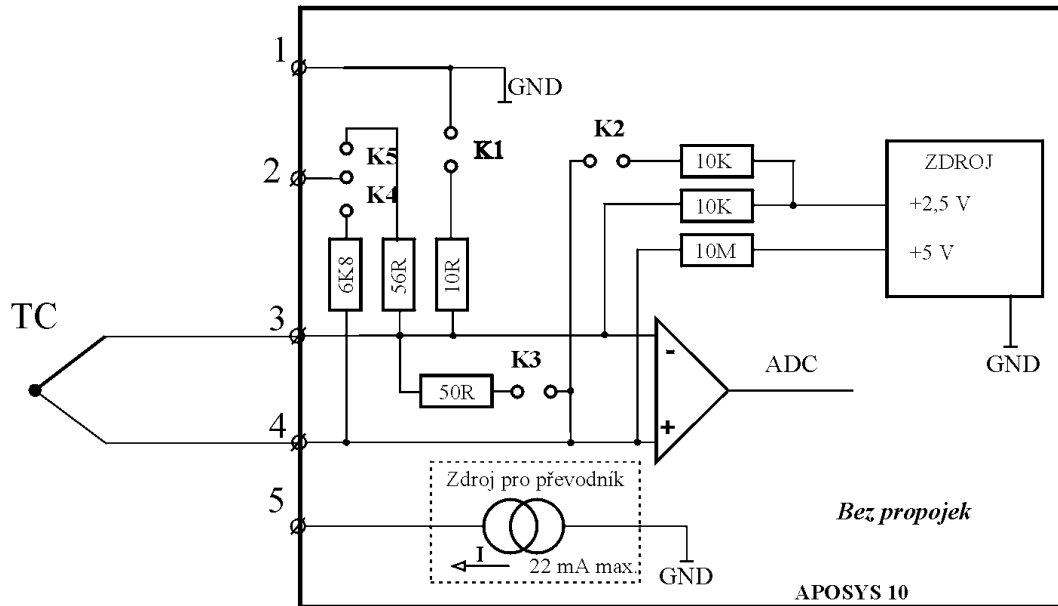
Připojení termočláčku
